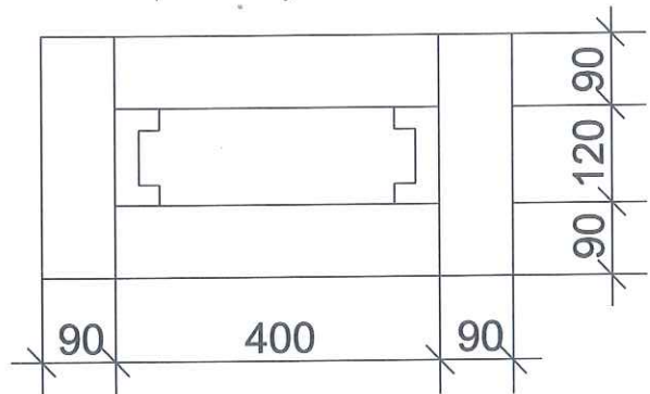
przekrój A-A
