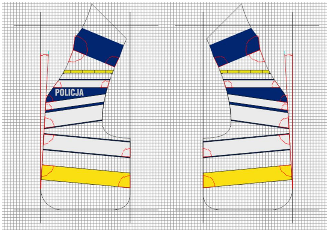
Rysunek 7. Graficzne przedstawienie odległości naszywania elementów odblaskowych i ich kąty nachylenia w przodzie kamizelki odblaskowej
