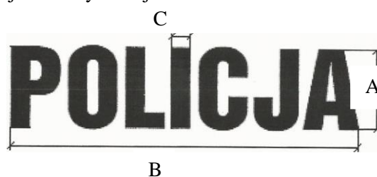
Rysunek 10. Napis „POLICJA” – wymiary
