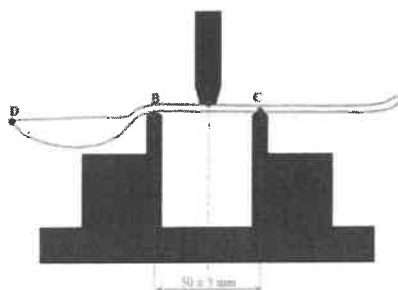
Rys.1. Sprawdzenie wytrzymałości sztućca – rysunek poglądowy
